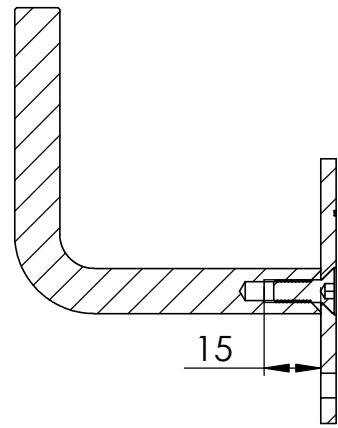
SCHNITT A-A
