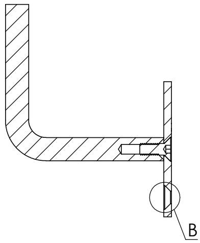
SCHNITT A-A
