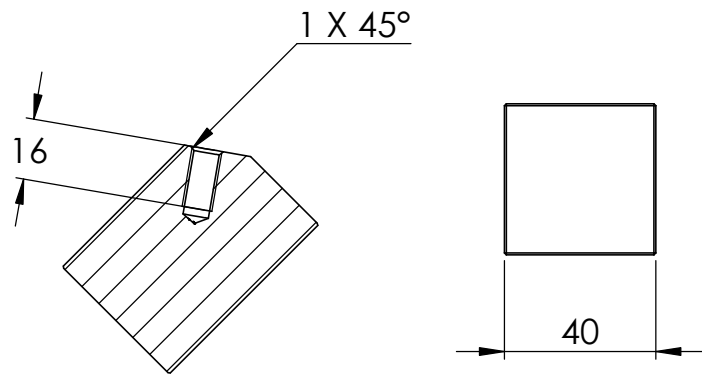
SCHNITT A-A
