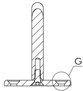
SCHNITT B-B
