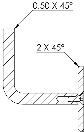
SCHNITT A-A
