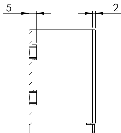
SCHNITT C-C
