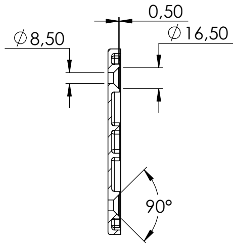
SCHNITT A-A
