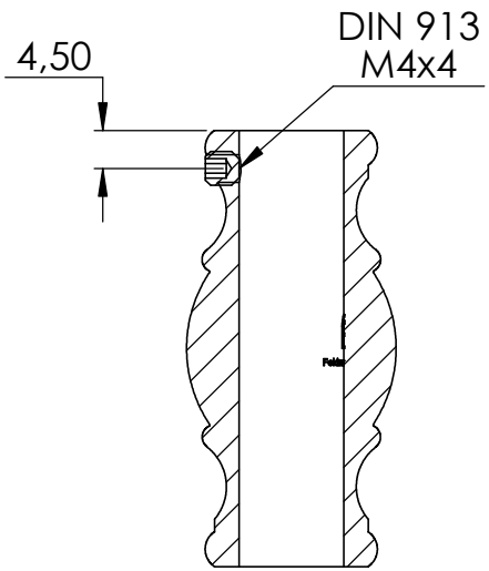
SCHNITT A-A
