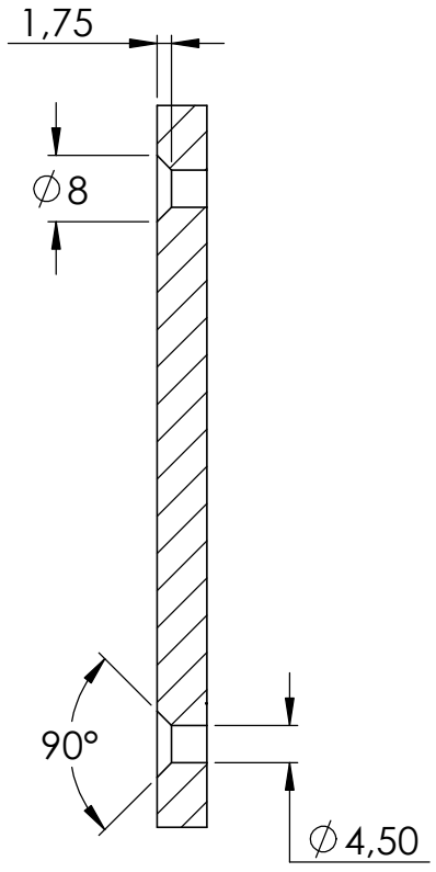
SCHNITT A-A
