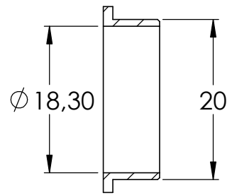
SCHNITT B-B
