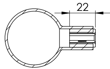
SCHNITT A-A
