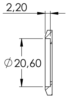
SCHNITT B-B
