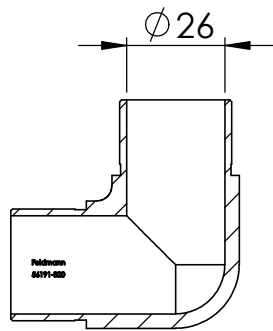
SCHNITT A-A
