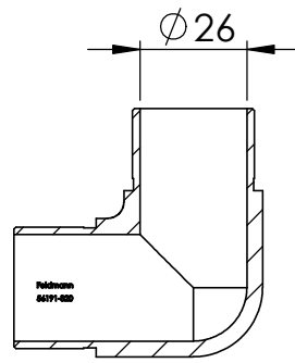
SCHNITT A-A
