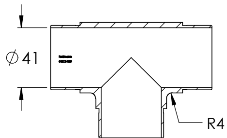
SCHNITT A-A
