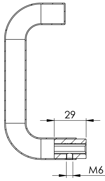
SCHNITT A-A
