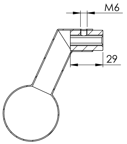
SCHNITT A-A
