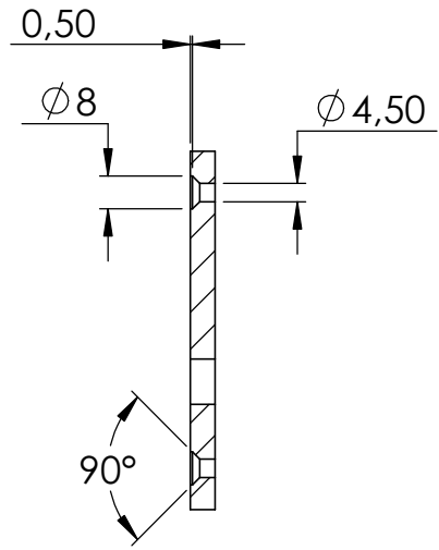
SCHNITT A-A
