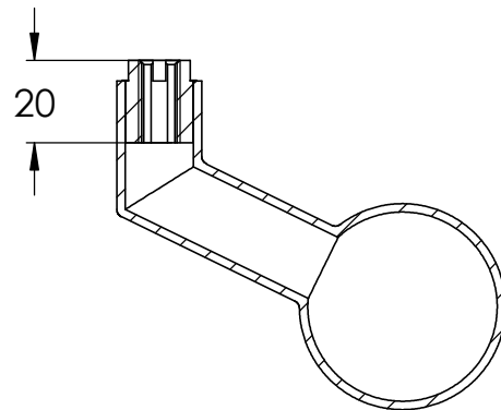
SCHNITT B-B
