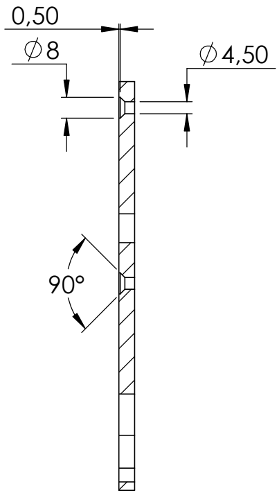
SCHNITT A-A
