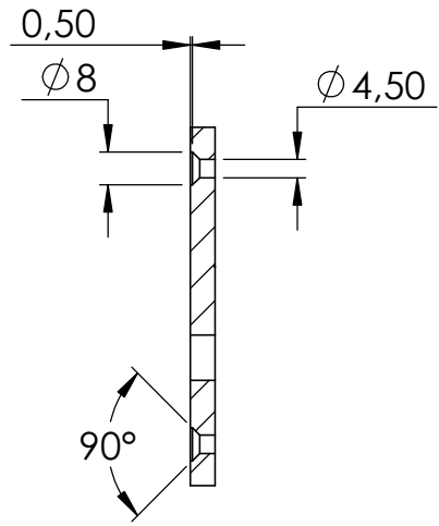
SCHNITT A-A
