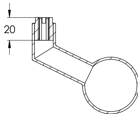
SCHNITT B-B
