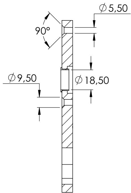
SCHNITT A-A
