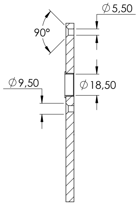
SCHNITT A-A
