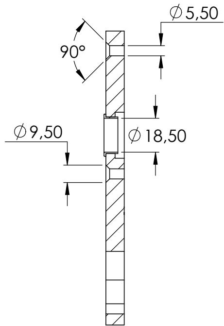
SCHNITT A-A
