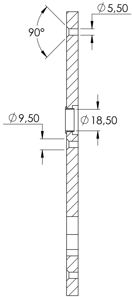
SCHNITT A-A
