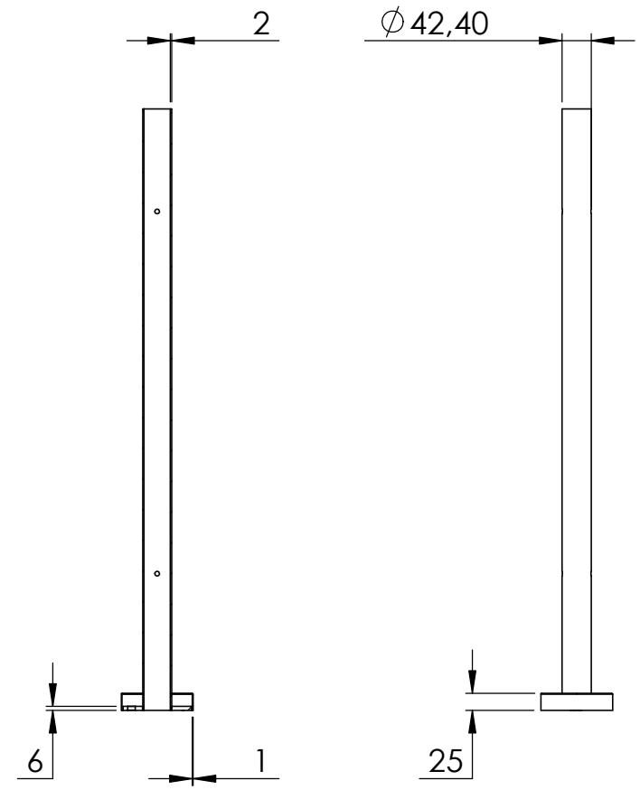
SCHNITT A-A
