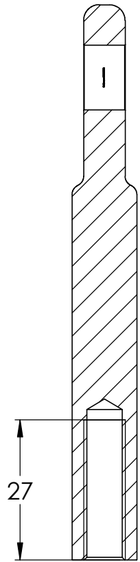
SCHNITT A-A
