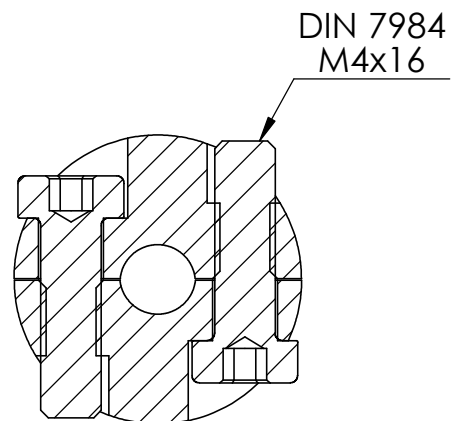
SCHNITT A-A
