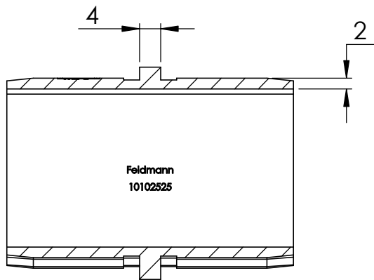
SCHNITT A-A
