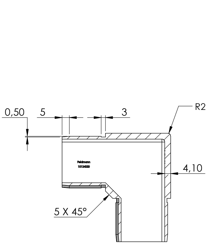
SCHNITT A-A
