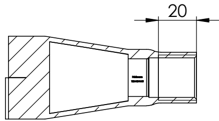
SCHNITT A-A
