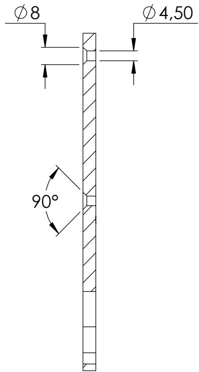
SCHNITT A-A
