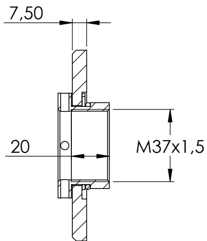
SCHNITT A-A
