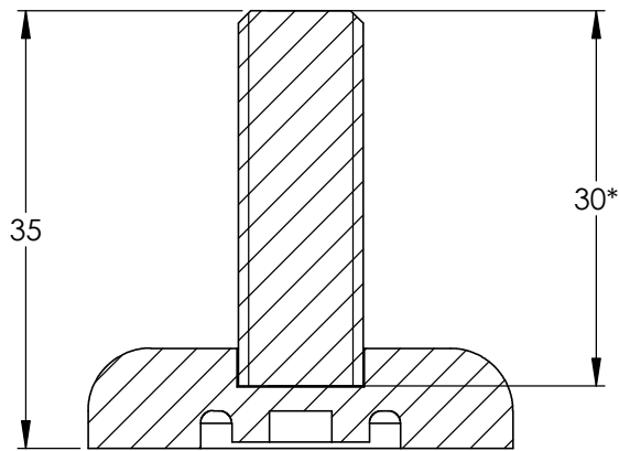
SCHNITT A-A
