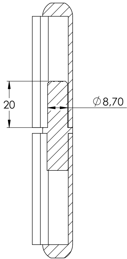
SCHNITT A-A
