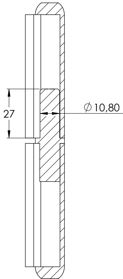
SCHNITT A-A
