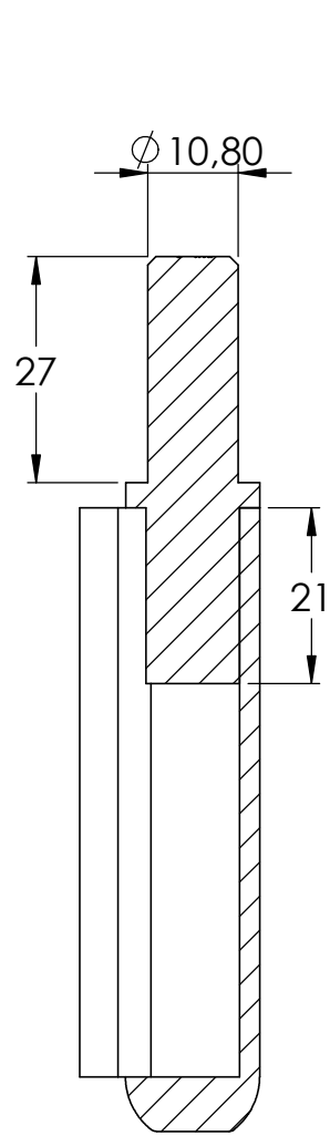
SCHNITT C-C
