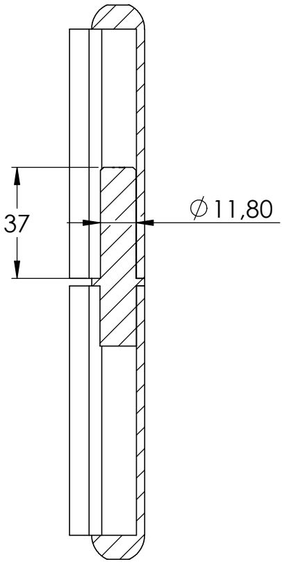
SCHNITT A-A
