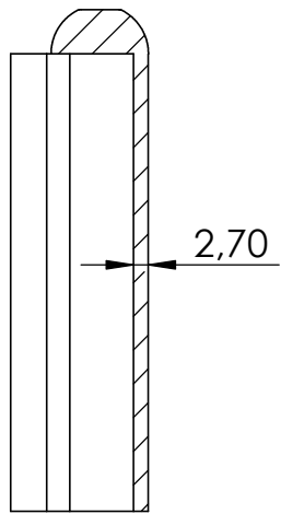
SCHNITT B-B
