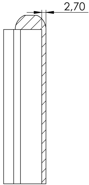
SCHNITT B-B
