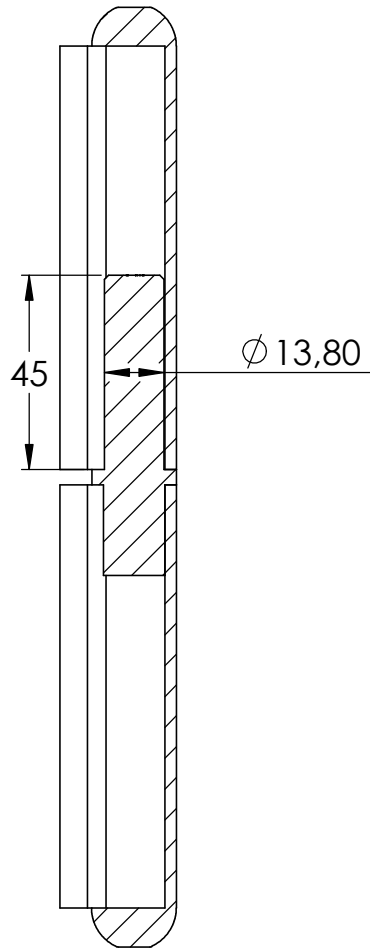
SCHNITT A-A
