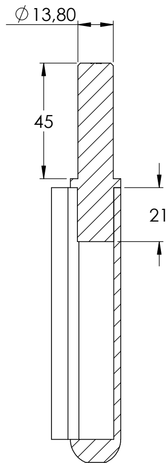
SCHNITT C-C
