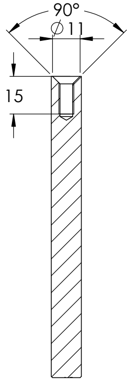
SCHNITT A-A
