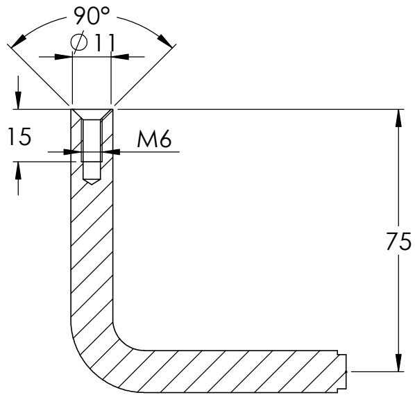
SCHNITT B-B
