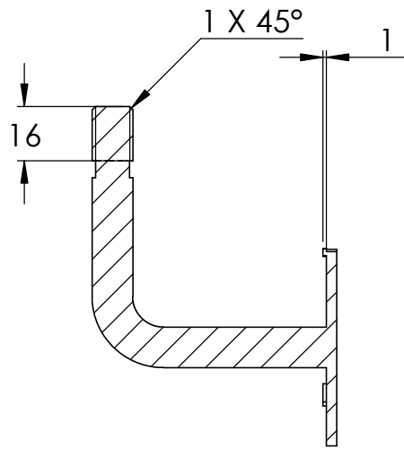
SCHNITT A-A
