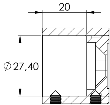
SCHNITT A-A
