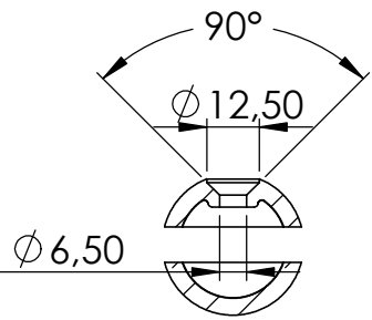
SCHNITT C-C
