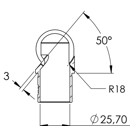
SCHNITT B-B
