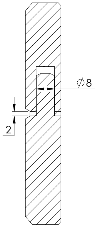
SCHNITT A-A
