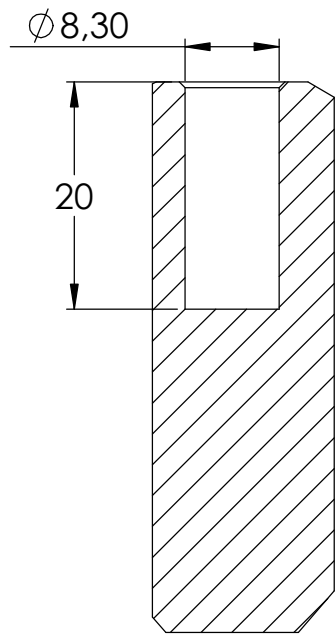
SCHNITT B-B
