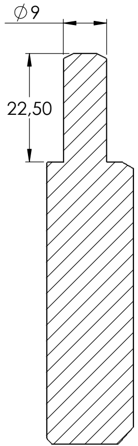
SCHNITT C-C
