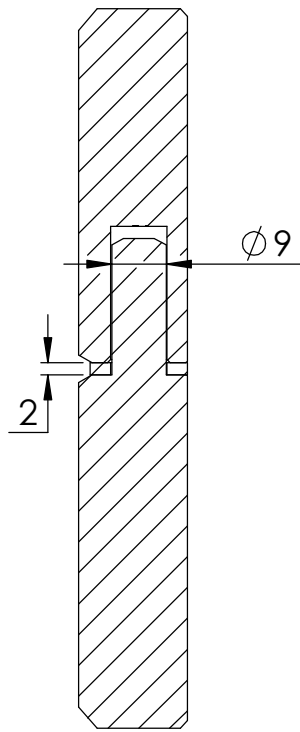
SCHNITT A-A
