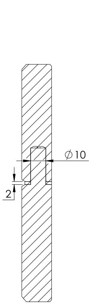
SCHNITT A-A
