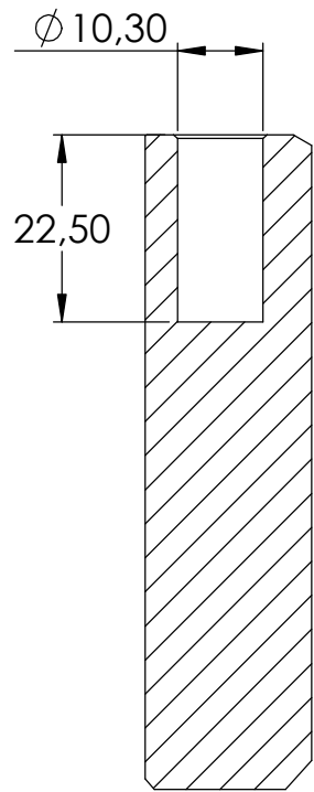
SCHNITT B-B
