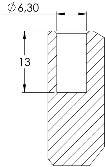
SCHNITT B-B
