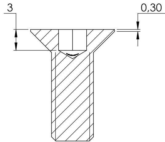
SCHNITT A-A
