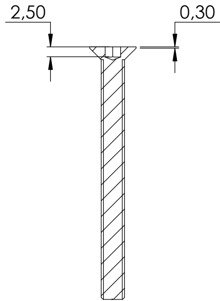
SCHNITT A-A
