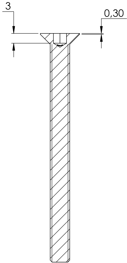
SCHNITT A-A
