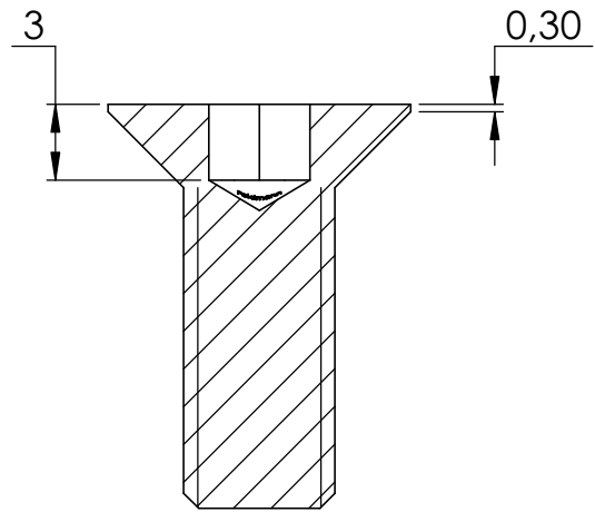
SCHNITT A-A
