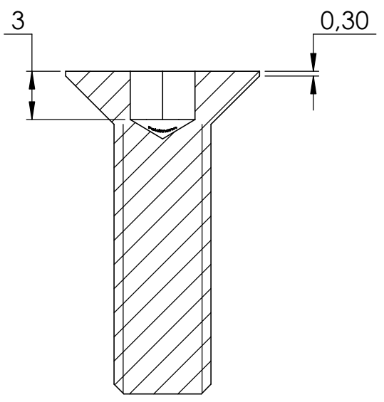
SCHNITT A-A
