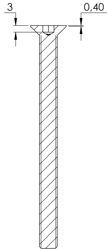
SCHNITT A-A
